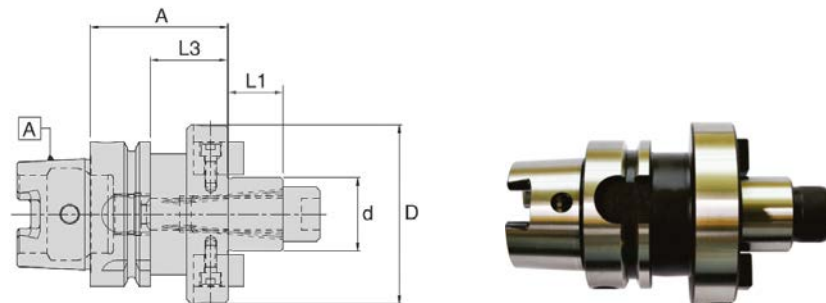
Aufnahme HSK-A100 für Aufsteckfräser Chuck HSK-A100 for face milling cutter
