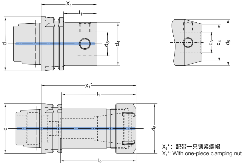
中心空腔 ER 40, 弹簧夹套刀柄 Collet chuck ER 40 with central bore
